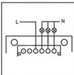
Odpojte napájení, připojte vodiče a utáhněte
