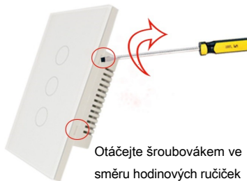
Jak otevřít vypínač v USA
